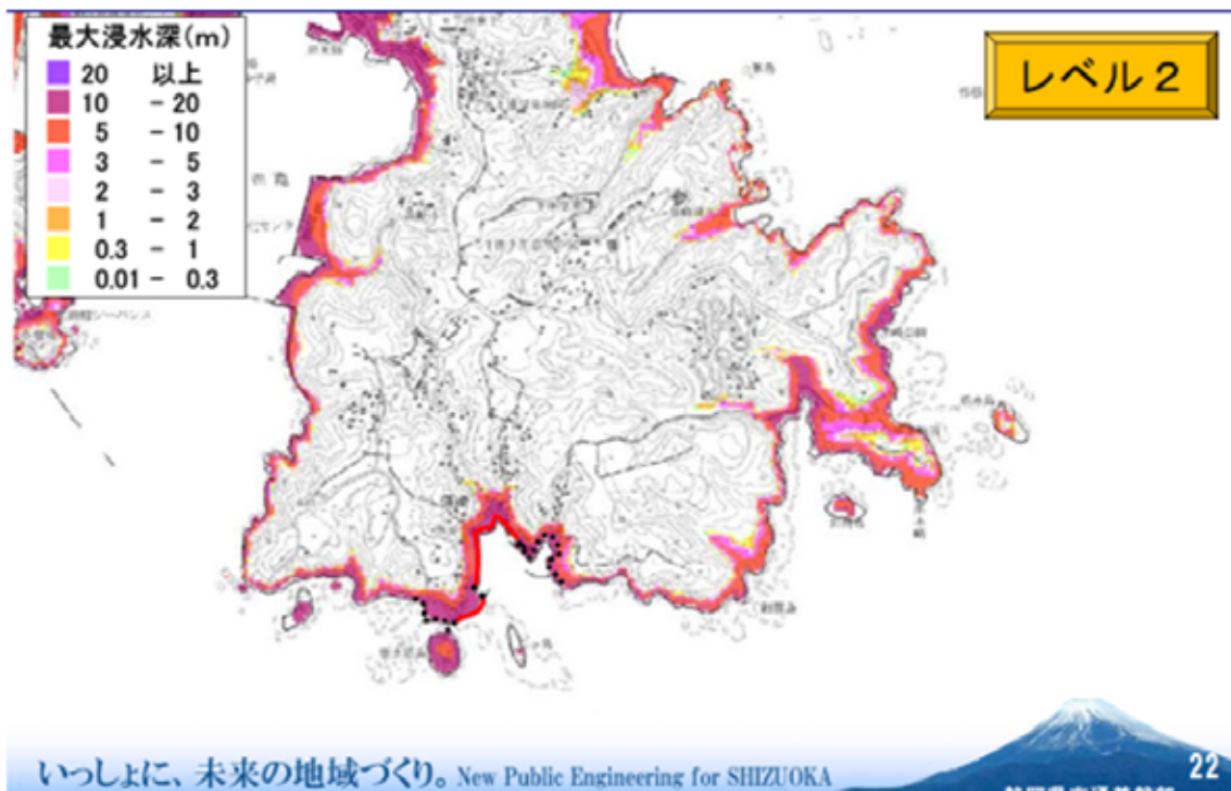
図2 須崎地区 南海トラフ沿いの最大クラスの地震（レベル2）最大浸水深図
