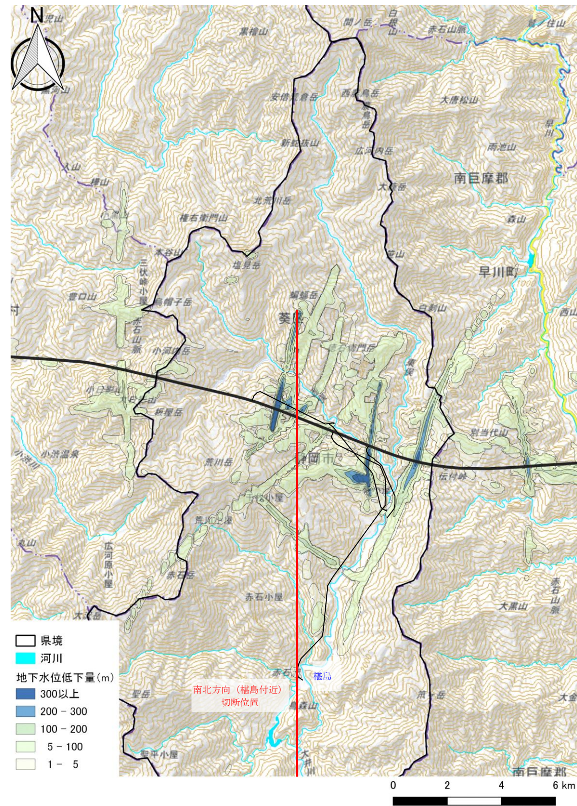
図 4.13 静岡市モデル 地下水位低下量平面図（トンネル掘削完了後恒常時）
