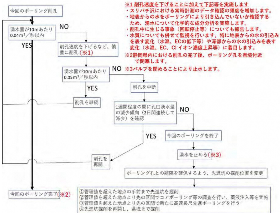
図 5 6 高速長尺先進ボーリングにおける調査中の管理フロー（更新）
