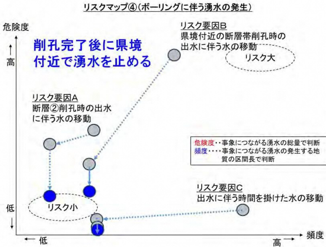
図 5 3 ポーリングに伴う湧水の発生に関わるリスクマップ④
