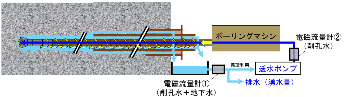
図 25 ボーリングにおける湧水量の測定方法 (高速長尺先進ボーリングの場合)
