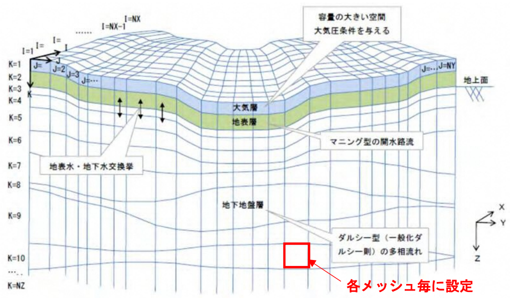
図 19 水収支解析モデル（静岡市モデル）
