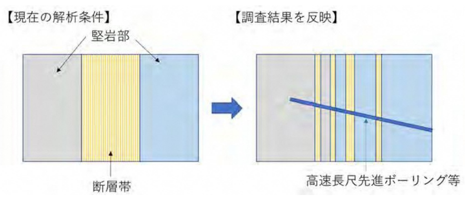
図 20 調査による地盤区分の把握のイメージ
