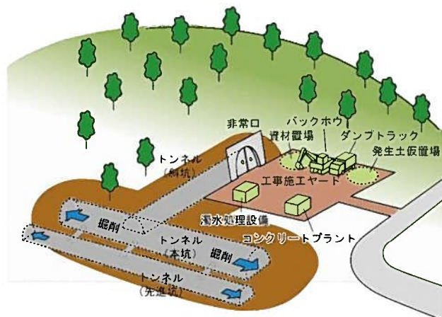
図6. 施工ヤードとトンネルの位置関係
