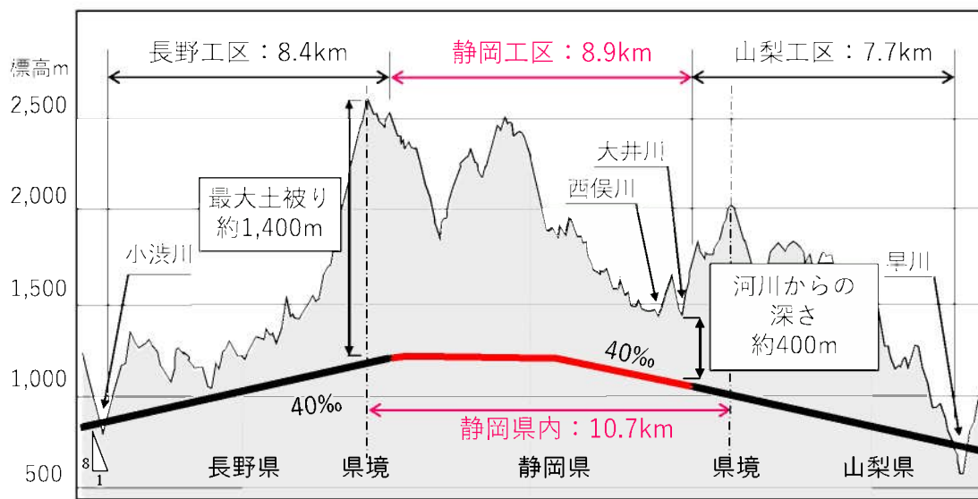
図3. トンネルの縦断図
