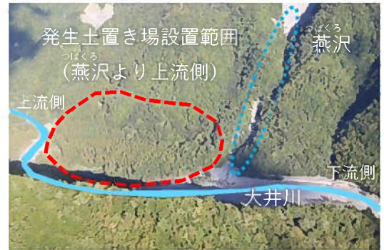
図30.燕沢付近発生土置き場の航空写真
