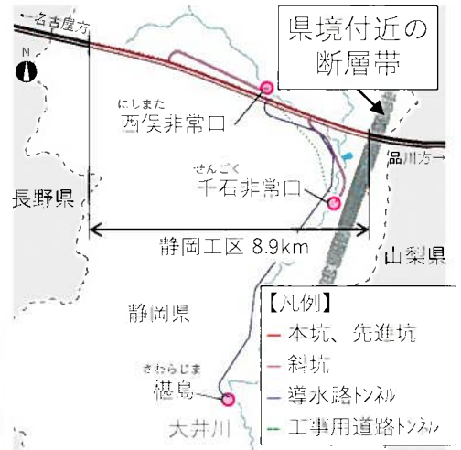
図14.県境付近の断層帯の位置図 (平面図)
