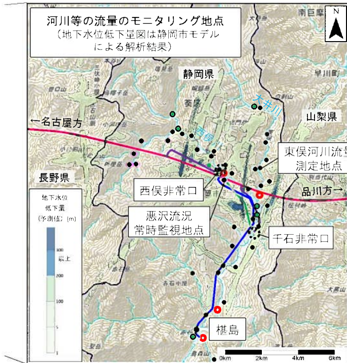
図36.上流部のモニタリング地点の例 (河川等の流量)
